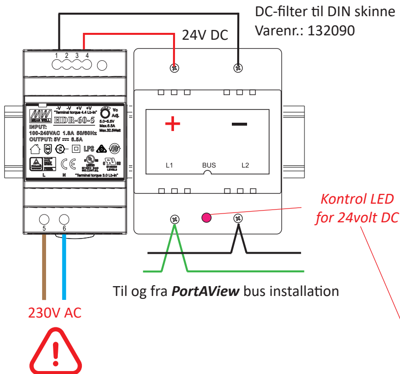
24V strømforsyning 2,5 A - 60 watt Varenr.: 132080
